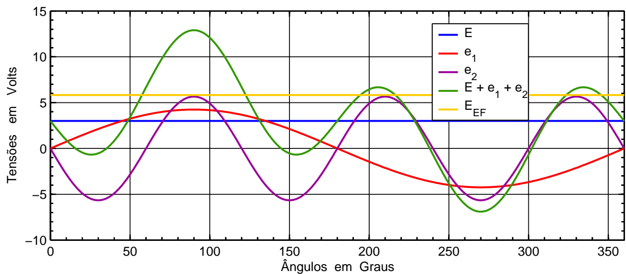
Fig. 10 – Tensão contínua com 3 V e componentes alternadas com 3 V EF e 4 V EF , e o triplo da frequência uma da outra.
